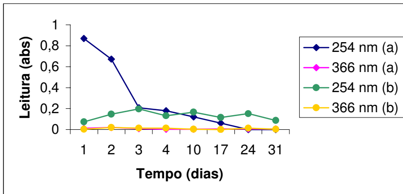
Figura 3. Produção de metabólitos por células de Parmotrema andinum imobilizadas em caulinita, utilizando acetato de sódio 1,0 mM. (a) extrato éter/acetato de etila; (b) extrato clorofórmio/acetonitrila
