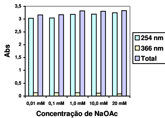
Figura 6. Produção total de substâncias fenólicas por células de P. andinum , imobilizadas em caulinita, utilizando acetato de sódio em diferentes concentrações
