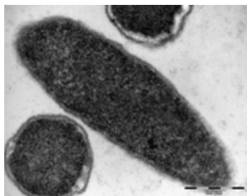
Figs.1 e 2. Bactéria E. coli resistente (ATCC 35218) em meio de cultura Mueller-Hinton líquido após 6 horas de incubação em 37°C.
