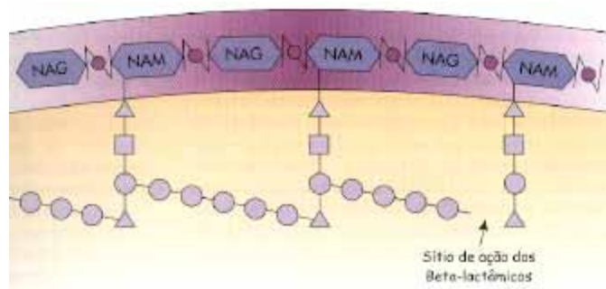
Figura 7. Mecanismo de ação dos antibióticos betalactâmicos (adaptado de Atlas, R.M., Principles of Microbiology, 1997)
