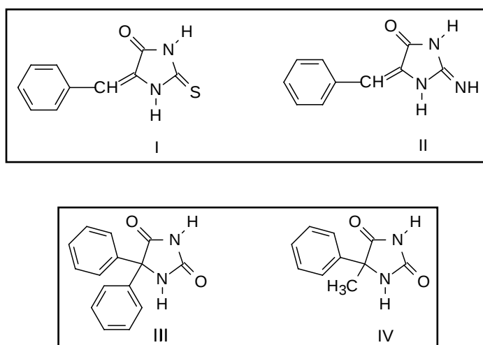
Figura 2. Estrutura química das imidazolidinas: (I) 5-benzilideno-2-tioxo-imidazolidina-4-ona, (II) 2-amino-5-benzilideno-imidazolidina-2,4-diona, (III) 5,5-difenil-imidazolidina-2,4-diona e (IV) 5-( p -clorofenil)-5-metil-imidazolidina-2,4-diona.
