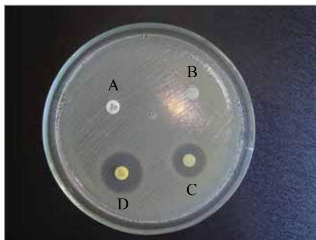
Fig.1 Sinergismo da imidazolidina sobre o antibiótico frente ao crescimento de E. coli resistente (ATCC35218). Em A, disco contendo ampicilina, em B, o solvente DMF, em C, disco impregnado com NN-41 e em D, a ação sinérgica do composto imidazolidínico sobre o antibiótico ampicilina.
