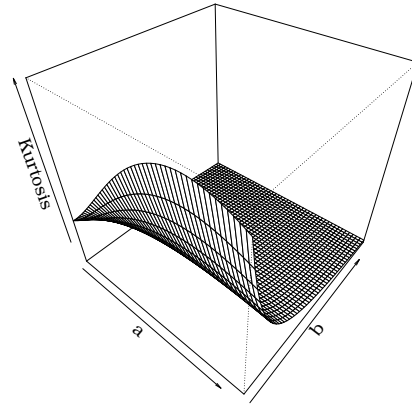
(d) \alpha = 0.1, \lambda = 1.5
