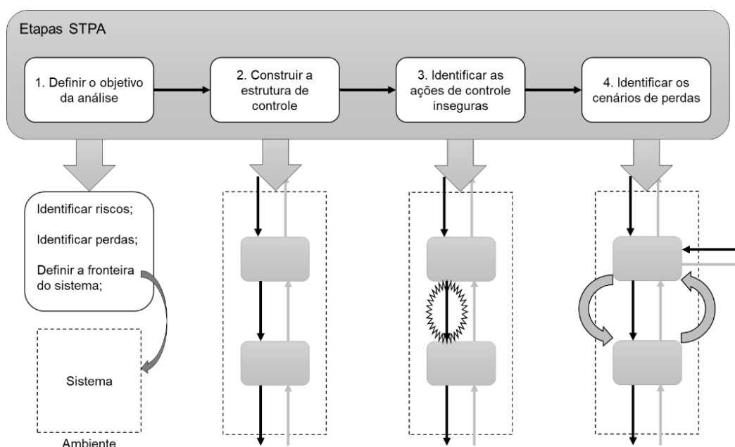
Figura 6 - Etapas básicas da técnica STPA
