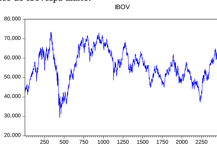
Gráfico 1 - Gráfico do Ibovespa diário.
