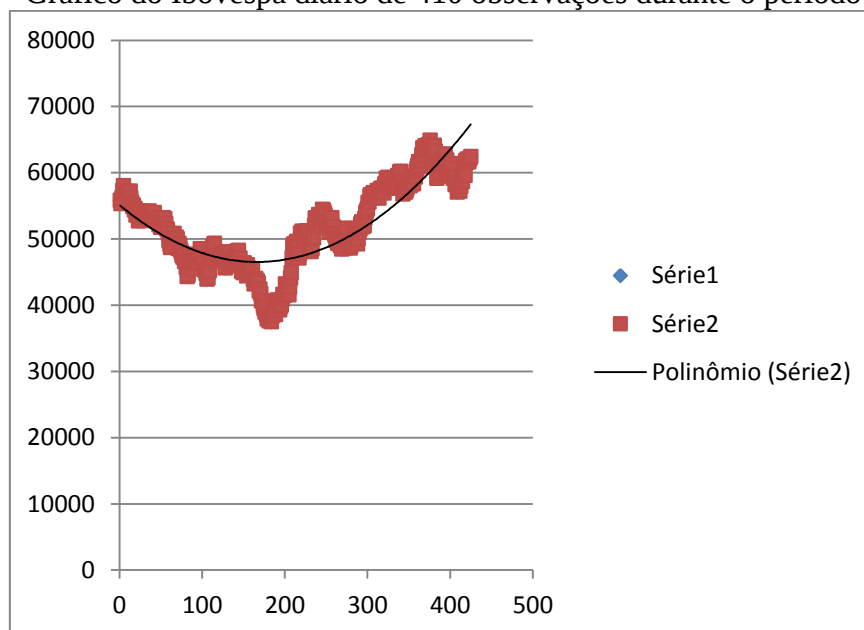
Gráfico 8 - Gráfico do Ibovespa diário de 410 observações durante o período proposto.
