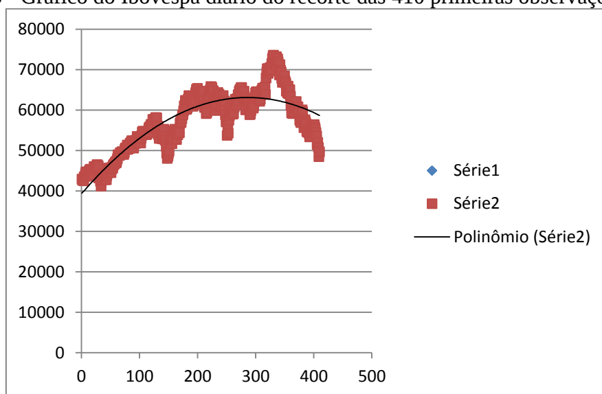
Gráfico 3 - Gráfico do Ibovespa diário do recorte das 410 primeiras observações.
