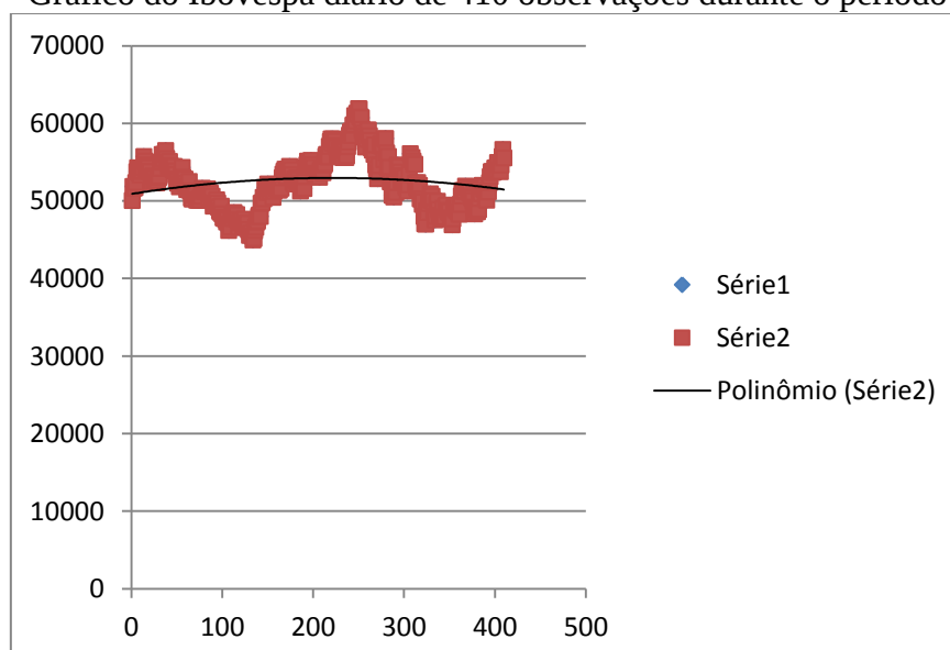
Gráfico 7 - Gráfico do Ibovespa diário de 410 observações durante o período proposto.
