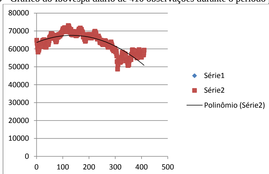
Gráfico 5 - Gráfico do Ibovespa diário de 410 observações durante o período proposto.
