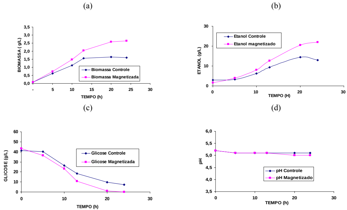
Figura 17 – Fermentação X 4 : curvas das variáveis monitoradas, na fermentação alcoólica por Saccharomyces cerevisiae , sem agitação mecânica, em função do tempo de fermentação: a – Biomassa (Peso seco), b – Produção de etanol, c – Consumo de glicose, d – Acompanhamento do pH.
