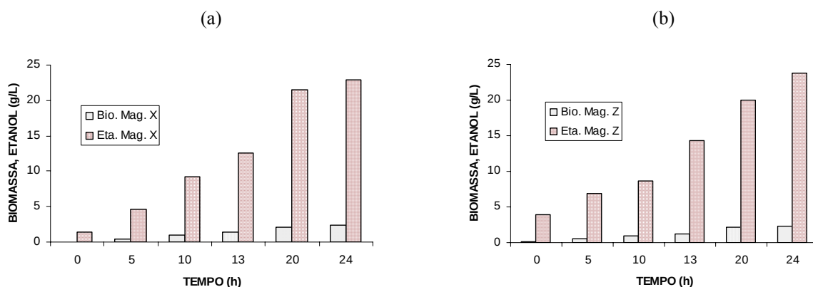
Figura 14 Gráficos dos valores médios da biomassa e etanol, nas fermentações alcoólicas por Saccharomyces cerevisiae , em função do tempo de fermentação. A – Biomassa e etanol fermentação X, b – Biomassa e etanol fermentação Z.
