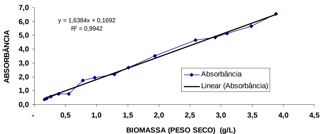
Figura 7 - Curva de calibração, absorbância, versus concentração celular
