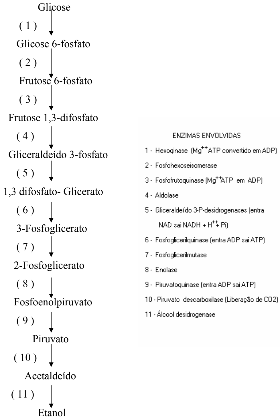
Figura 1 - Degradação da glicose (Via de Embden-Meyerhof-Parnas)
