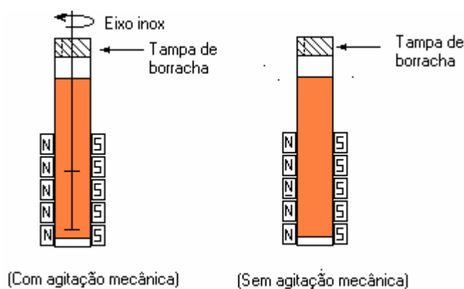
Figura 5 - Arranjo 1 dos biorreatores expostos a campo magnético gerado por magnetos cilíndricos
