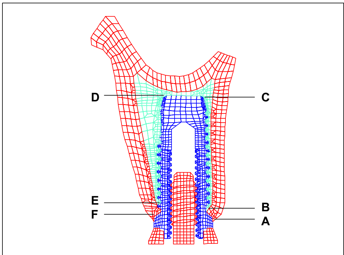
Figura 4: Elementos investigados em cada região.
