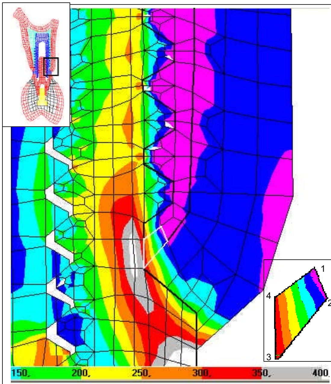
Figura 12: Tensões de Von Missses (MPa) na região B do modelo 4. O elemento (1524) em destaque foi investigado em seus 4 nós.
