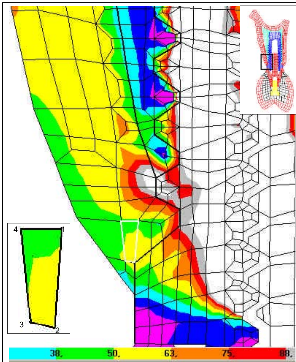
Figura 8: Tensões de Von Missses (MPa) na região F do modelo 4. O elemento (1874) em destaque foi investigado em seus 4 nós.
