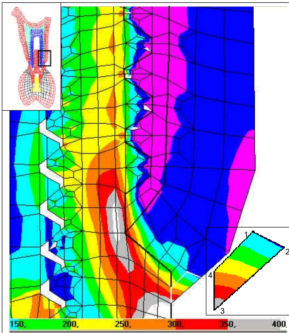
Figura 13: Tensões de Von Missses (MPa) na região A do modelo 4. O elemento (2084) em destaque foi investigado em seus 4 nós.
