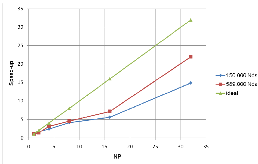
Figura 5.15 – Comparação entre curvas de speed-up para o um mesmo problema tratado com malhas de tamanhos diferentes.
