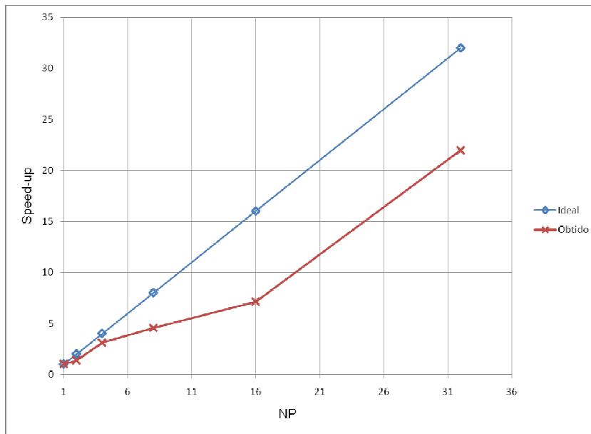
Figura 5.12 – Comparação entre as curvas de speed-up ideal e real para a malha de 589.487 nós.
