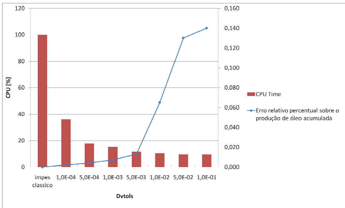
Figura 4.12 – Relação entre o tempo total de CPU e a acurácia dos resultados para vários DVTOL. É tomada como referência a curva de óleo acumulado do método IMPES tradicional. Apenas para a malha de 10.448 nós com meio heterogêneo
