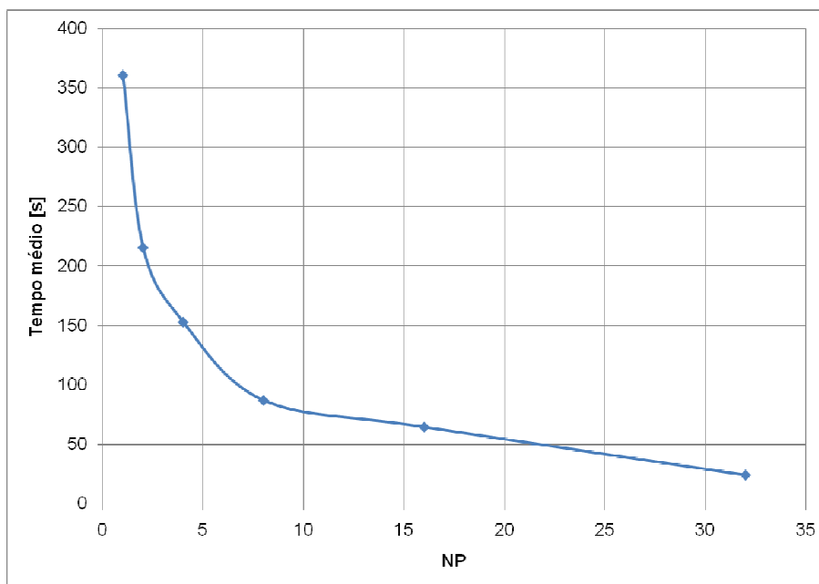
Figura 5.11 – Redução do tempo médio de execução por passo de tempo para a malha de 150.725 nós.
