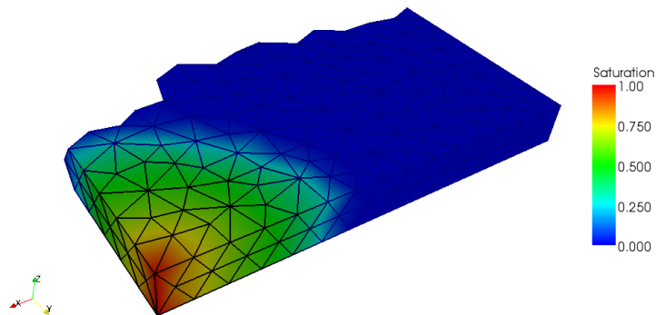
Figura 5.7 – Partição de uma malha mostrando o campo de saturação de água em um dado instante da simulação.
