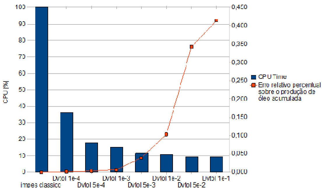
Figura 4.5 – Relação entre o tempo total de CPU e a acurácia dos resultados para vários DVTOL. É tomada como referência a curva de óleo acumulado do método IMPES tradicional. Apenas para a malha de 10.201 nós com meio homogêneo.
