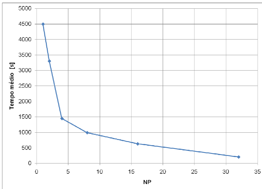
Figura 5.13 – Redução do tempo médio de execução por passo de tempo para a malha de 589.487 nós.
