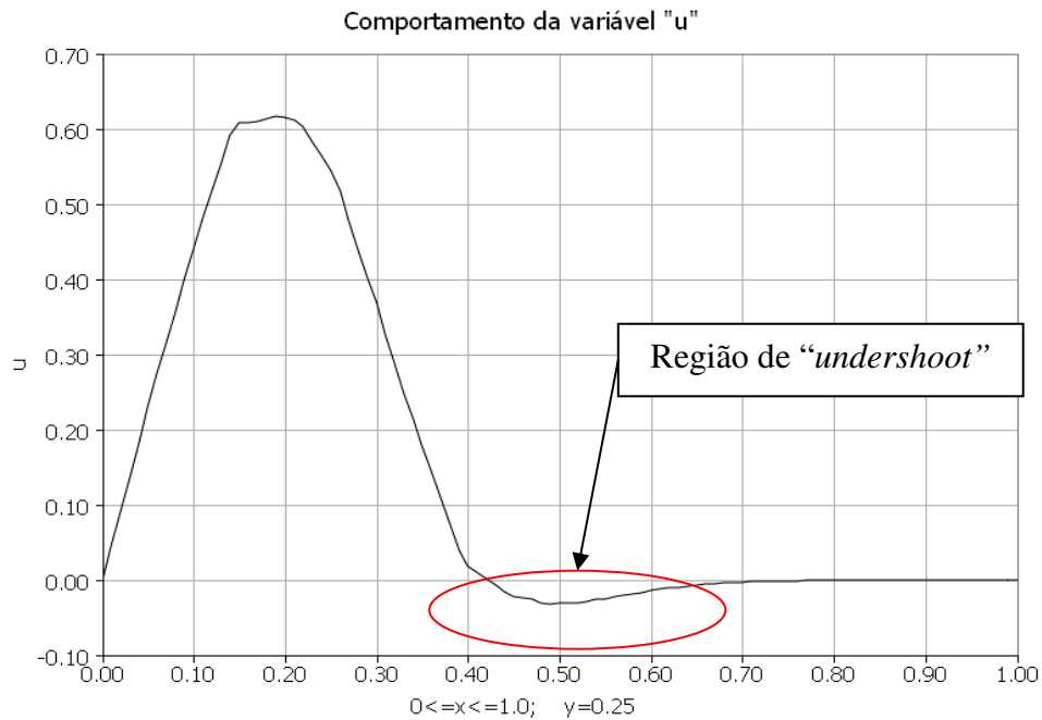
Figura 3.8 – Comportamento da variável u ao longo de uma reta paralela ao eixo x passando pelo centro do domínio. Para um problema com valores prescritos mínimo e máximo de 0.0 e 2.0, respectivamente, esperava-se que os resultados ficassem confinados dentro desse intervalo. Devido a forte anisotropia, verifica-se a presença de “ undershoots ”, ou seja, valores calculados abaixo do mínimo esperado.
