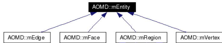
Figura 5.3 – Diagrama de classes para mEntity .
