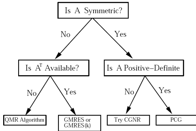
Figura 5.5 – Possível árvore de decisões na escolha do método iterativo para problemas de grande porte e não deve ser tratada como uma regra única.
