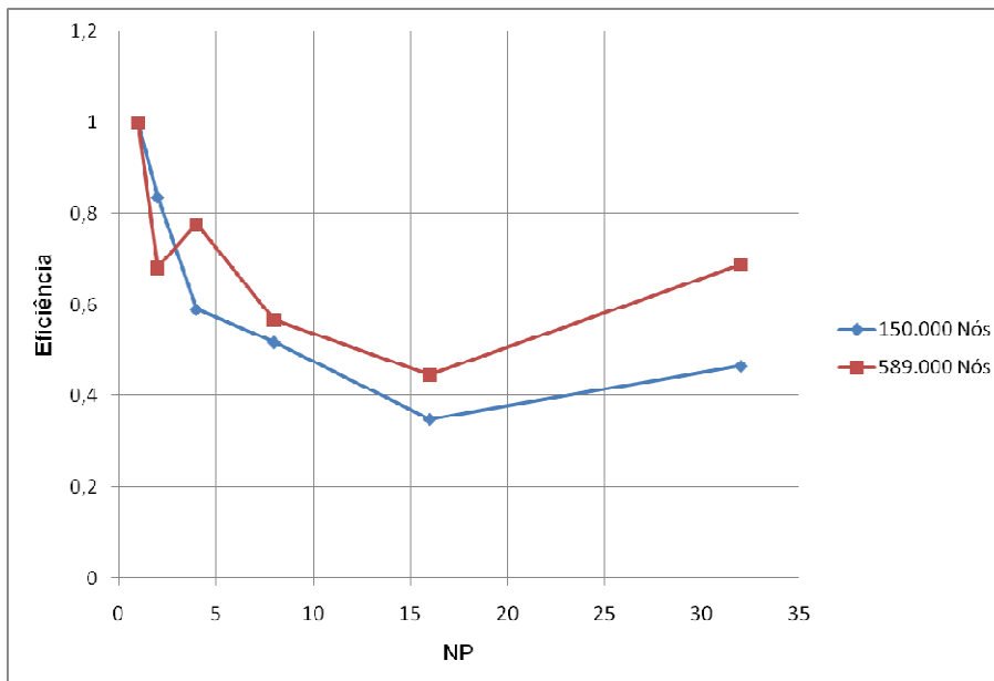
Figura 5.14 – Comparação das curvas de eficiência para duas malhas.
