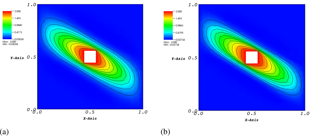
Figura 3.7 – Solução numérica para o problema homogêneo e anisotrópico com solução não suave: ângulo de rotação \theta = 5\pi/6 ; a) EBFV1; b) EBFV2.
