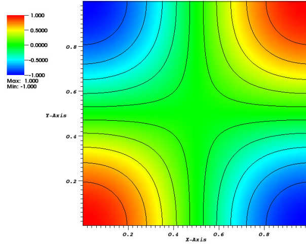
Figura 3.2 – Equação elíptica com coeficientes isotrópicos e contínuos: campo escalar u obtido com o EBFV2 usando uma malha triangular (65x65).
