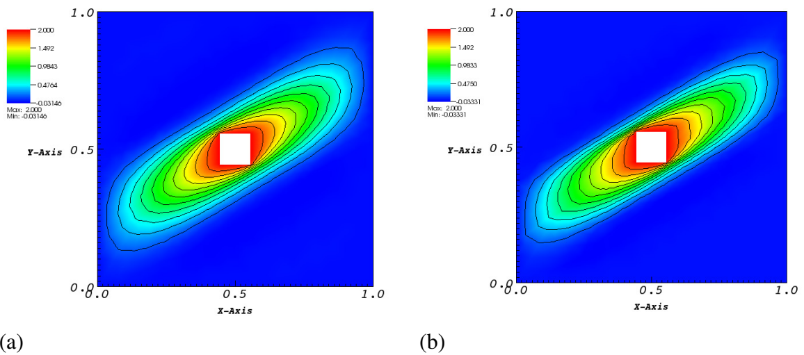
Figura 3.6 – Solução numérica para o problema homogêneo e anisotrópico com solução não suave: ângulo de rotação \theta = \pi/6 ; a) EBFV1; b) EBFV2.
