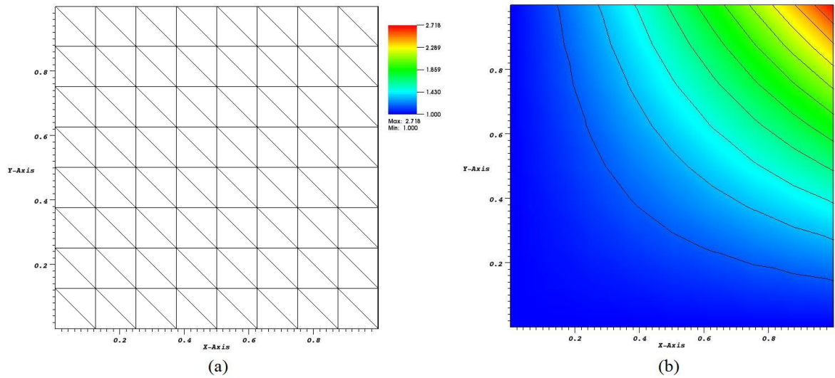
Figura 3.3 – Meio homogêneo e anisotrópico: a) malha triangular (9x9); b) campo escalar u obtido com o EBFV1.
