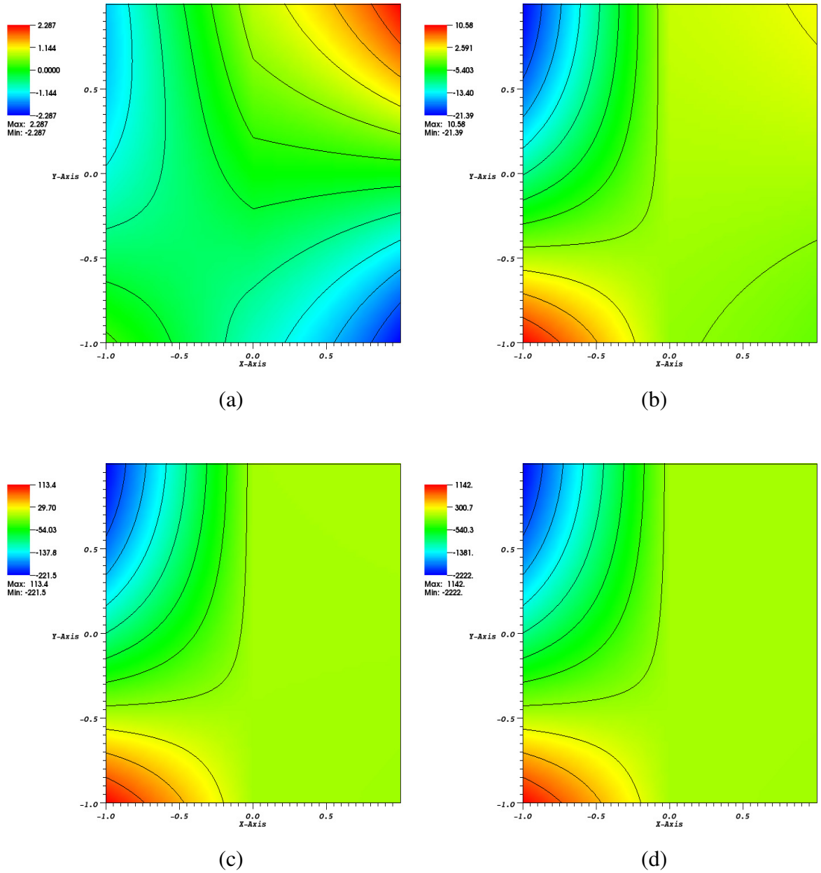
Figura 3.4 – Linhas de contorno da função escalar u(x, y) obtidas com o EBFV1 usando uma malha estruturada triangular (65x65) para diferentes valores de \alpha : (a) \alpha = 1.0 ; (b); \alpha = 10.0 (c) \alpha = 100.0 ; (d) \alpha = 1000.0
