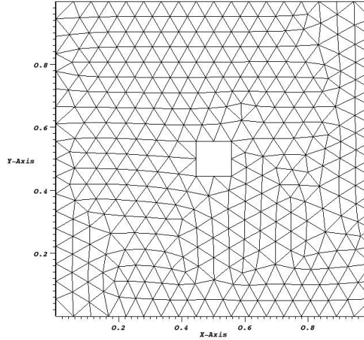
Figura 3.5 – Geometria e malha triangular não-estruturada usada para resolver o problema homogêneo e anisotrópico com solução não suave.
