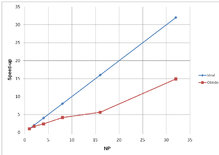
Figura 5.10 – Comparação entre as curvas de speed-up ideal e real para a malha de 150.725 nós.
