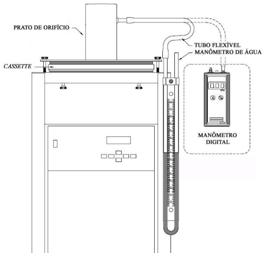
Figura 11 – Esquema do processo de calibração do Hivol HVS 3000.
