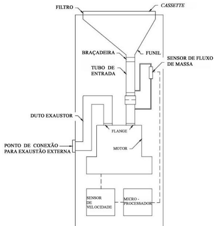
(c) Corpo do Hivol .
