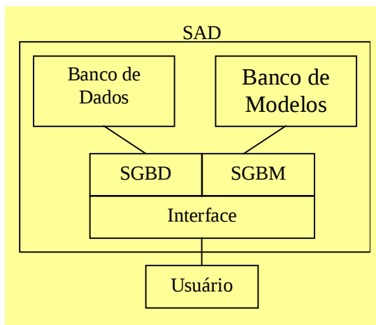
Figura 2.11 - Componentes de um SAD Fonte: Sprague e Watson (1991)
