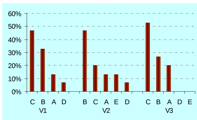
Figura 5.8 – Ocorrências das variáveis originais no Fator 1 para decisores
