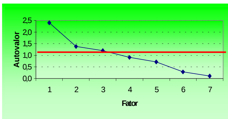
Figura 5.1 – Autovalores para profissionais de TI
