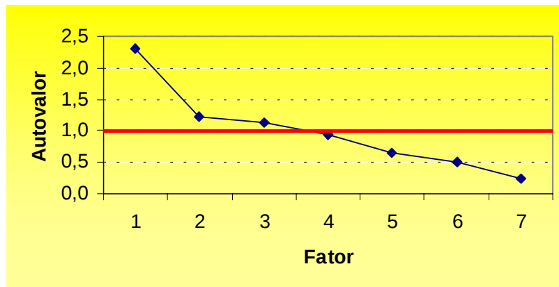
Figura 5.6 – Autovalores para decisores
