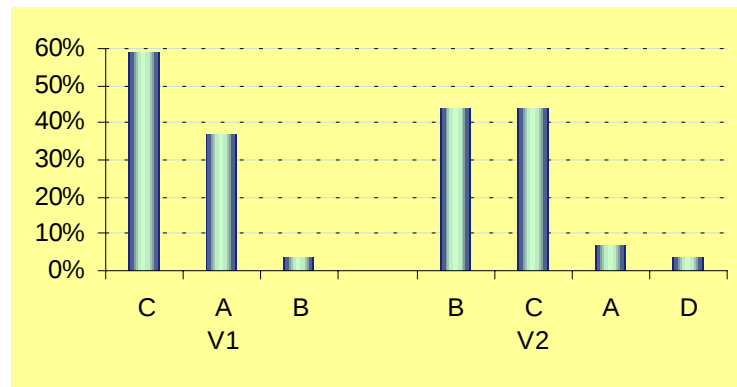
Figura 5.4 – Ocorrências das variáveis originais no Fator 2 para profissionais de TI
