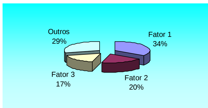
Figura 5.2 – Percentagem de variância explicada pelos fatores para profissionais de TI
