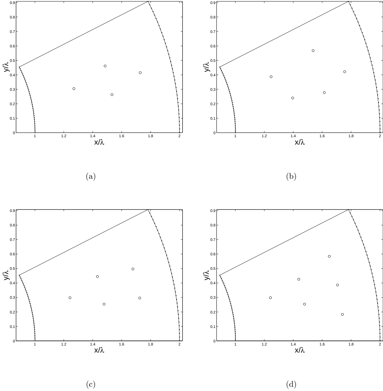
Figura 4.8: Posicionamento de vórtices no interior de um supercondutor. Os vórtices se posicionam de forma a minimizar a energia livre de Gibbs. As posições foram obtidas numericamente. Os parâmetros utilizados foram: a = \lambda , b = 2\lambda \beta = 0.2\pi . Os valores de campo H , em unidades de \Phi_0/\lambda^2 , atribuídos no sentido horário a partir do canto superior esquerdo, são: 0.56, 0.59, 0.67 e 0.77
