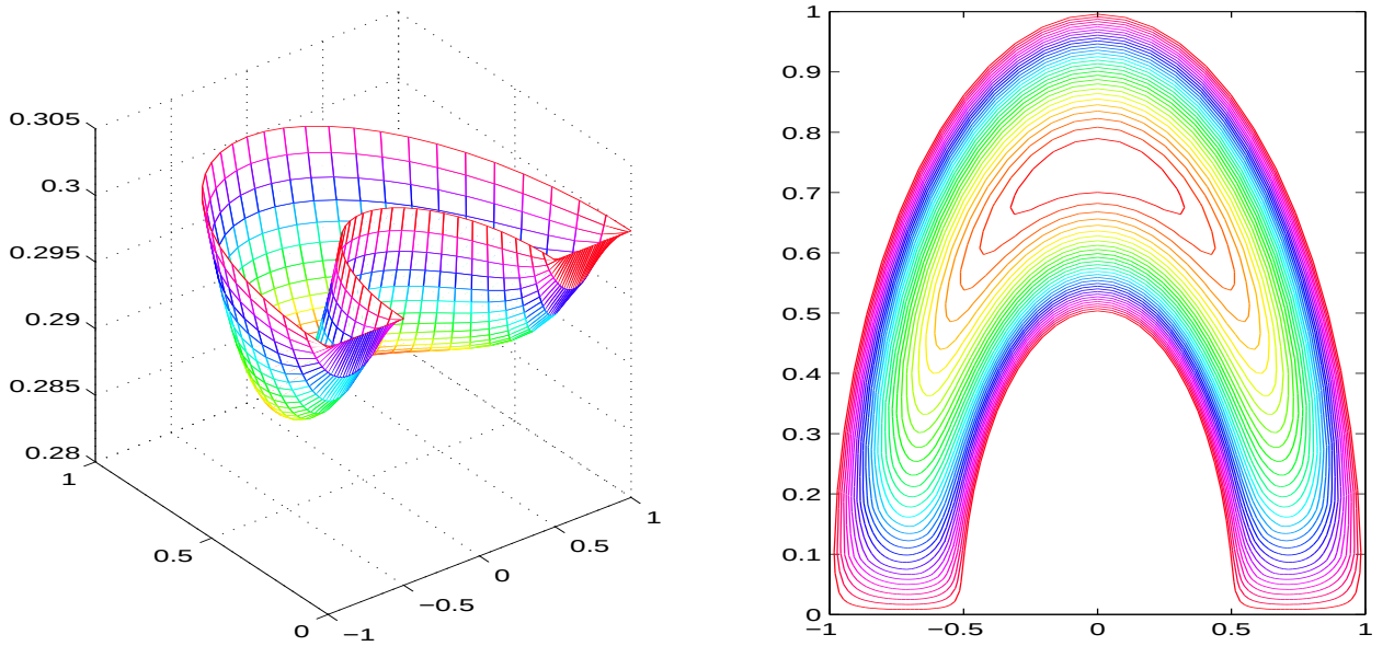
Figura 4.3: Campo Meissner de um supercondutor semi-infinito com uma indentação em um campo externo aplicado paralelamente à superfície do material. À esquerda temos o campo Meissner, h_M , e à direita sua curva de nível. Os parâmetros utilizados foram a = 0.5\lambda , b = \lambda e \beta = \pi .
