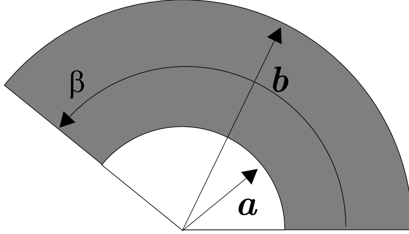
Figura 4.1: Sistema confinado. O supercondutor ocupa a região escura compreendida no intervalo a \leq \rho \leq b e 0 \leq \phi \leq \beta . a é o raio interno, b é o raio externo. O ângulo de corte \beta pode variar de zero até 2\pi . O campo H externo está paralelo ao eixo do cilindro na direção \hat{z} saindo na página.
