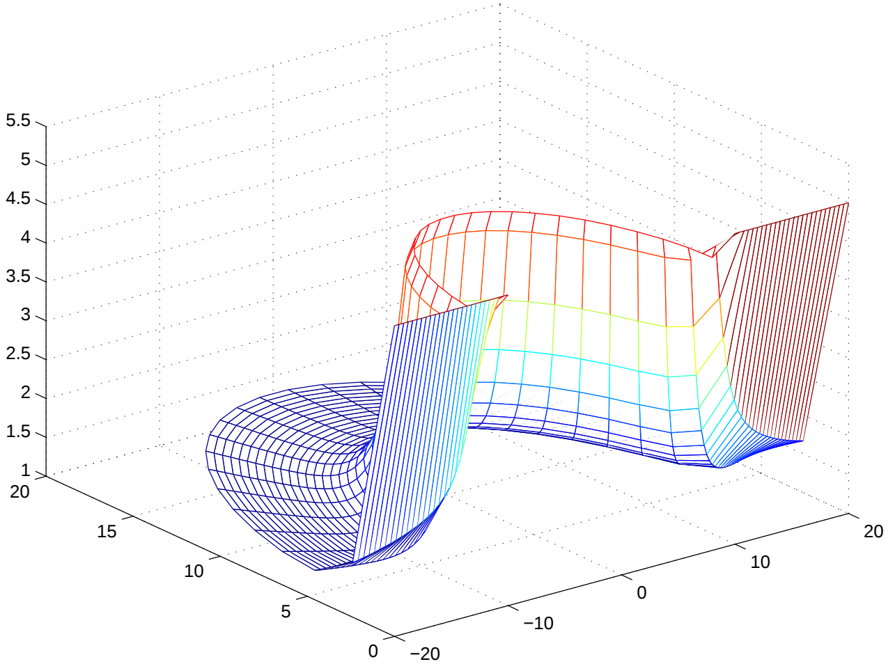
Figura 3.11: Energia livre de um supercondutor semi-infinito com uma indentação em função da posição de um vórtice no interior do meio. O material encontra-se no estado misto do supercondutores tipo-II. Os parâmetros utilizados foram: N = 1 , a = 0.5\lambda , \beta = \pi e H = 5 \frac{\phi_0}{\lambda^2} .
