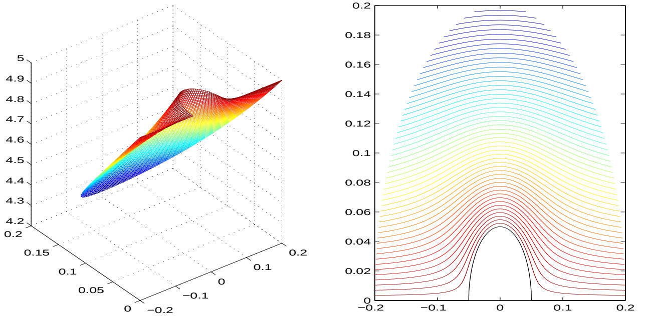
Figura 3.10: Campo Meissner de um supercondutor semi-infinito com uma indentação na presença de uma campo externo paralelo a superfície, no regime em que \lambda \gg a . À esquerda temos o campo obtido pela equação 3.46 e à direita suas curvas de nível. Os parâmetros utilizados foram : N = 1 , a = 0,05\lambda , \beta=\pi e H = 5\frac{\phi_0}{\lambda^2} .
