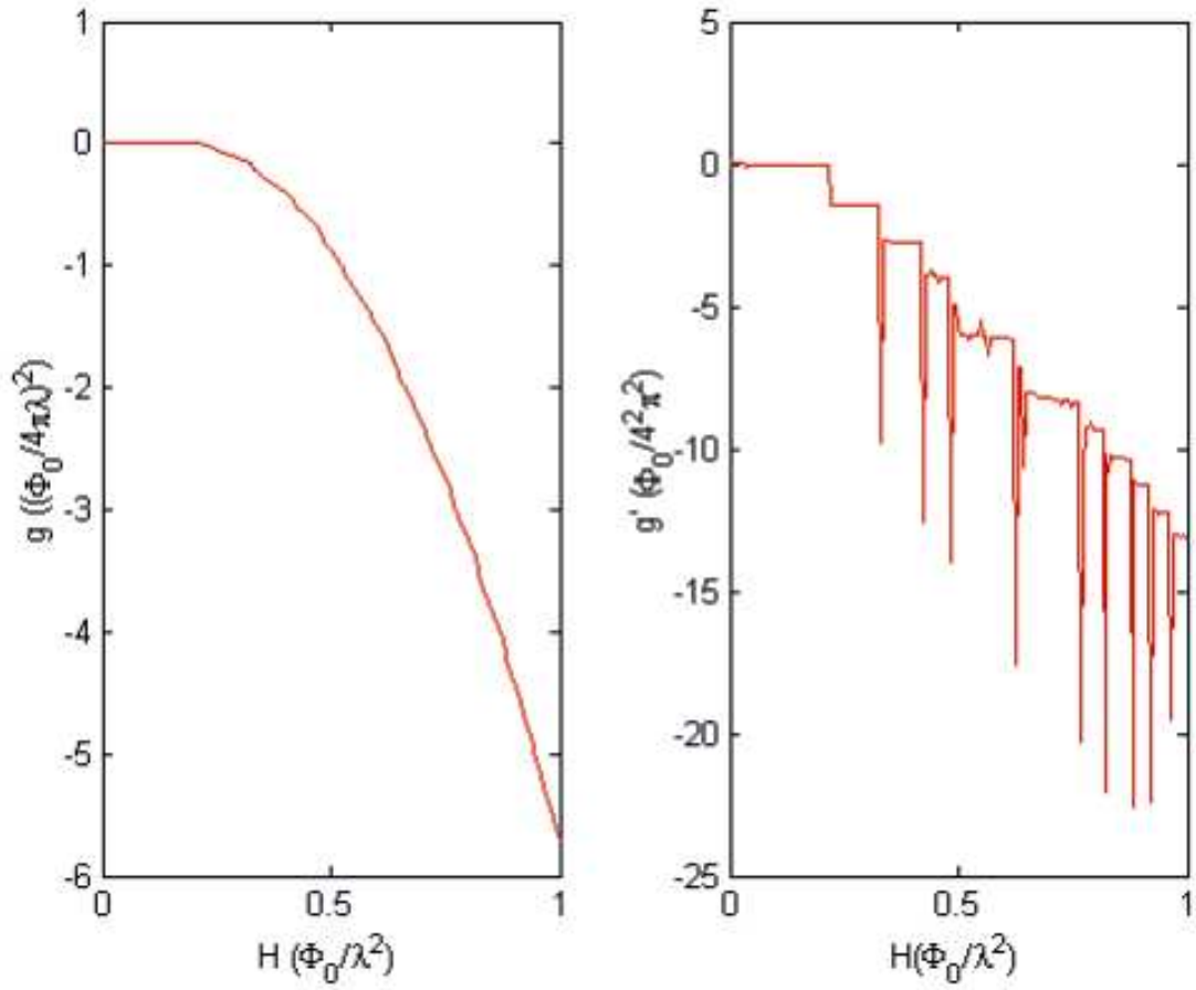
Figura 4.4: Energia de equilíbrio do sistema. Os parâmetros utilizados foram: a = \lambda , b = 2\lambda e \beta = 0.3\pi . O campo H está variando de 0 até 1.1, com um incremento de 0.001. Estamos considerando apenas os termos associados ao sistema de vórtices: A energia de interação, a auto energia e a interação do campo externo com os vórtices.
