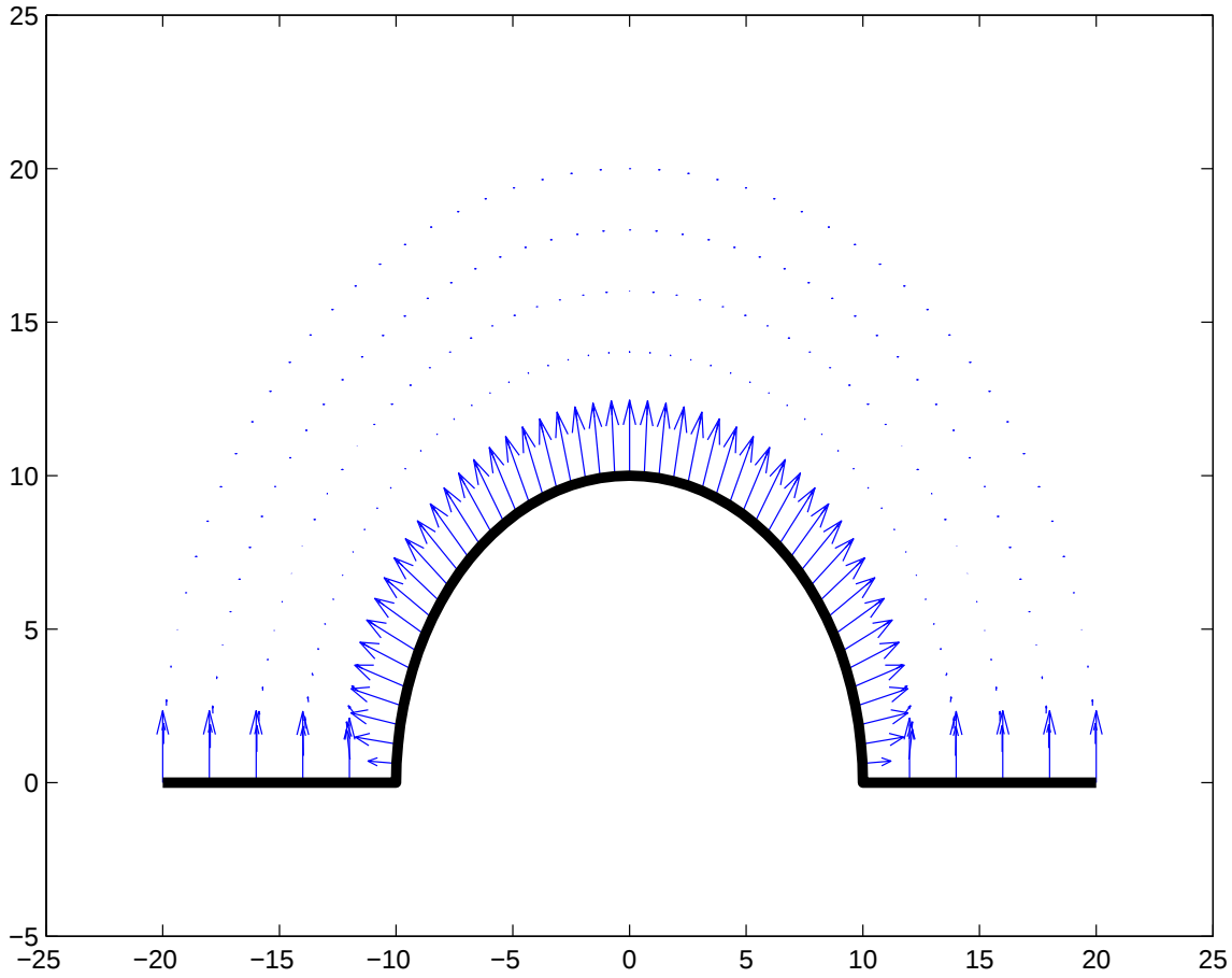
Figura 3.13: Força sofrida por um vórtice devido a presença do campo magnético externo em um supercondutor semi-infinito com uma indentação na superfície. As setas indicam que a força Meissner direciona os vórtices para o interior do material. Os parâmetros utilizados foram: a = \lambda , e H = 5 \frac{\phi_0}{\lambda^2} .
