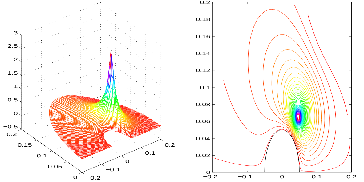
Figura 3.9: Auto-campo magnético em um supercondutor com uma indentação na superfície contendo um vórtice no interior no regime em que \lambda \gg a . À esquerda nós temos o auto-campo (3.44) e à direita suas curvas de nível. Os parâmetros utilizados foram : N = 1 , a = 0,05\lambda , \beta=\pi e \xi = 0,1\lambda .
