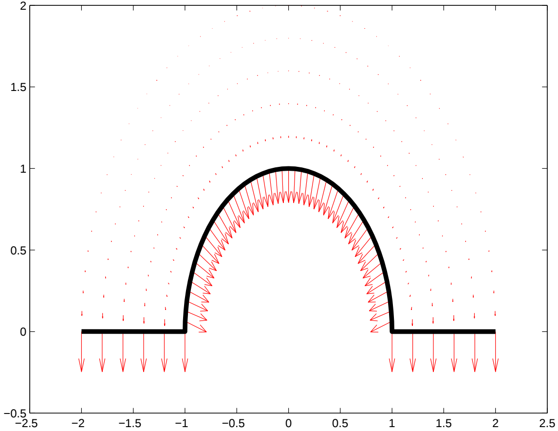
Figura 3.12: Força sofrida por um vórtice devido à interação atrativa com as suas imagens na ausência de campo externo. Os vetores representam a força descrita na equação 3.60. Os parâmetros envolvidos foram: a = \lambda , e \xi = \lambda/60
