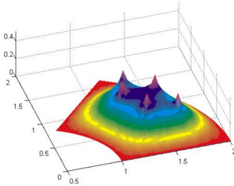
Figura 4.2: Auto-magnético no interior de um supercondutor tipo-II no estado misto contendo cinco vórtices no seu interior. Os parâmetros utilizados foram: a = \lambda , b = 2\lambda e \beta = 0.3\pi . As cores indicam curvas equipotenciais.
