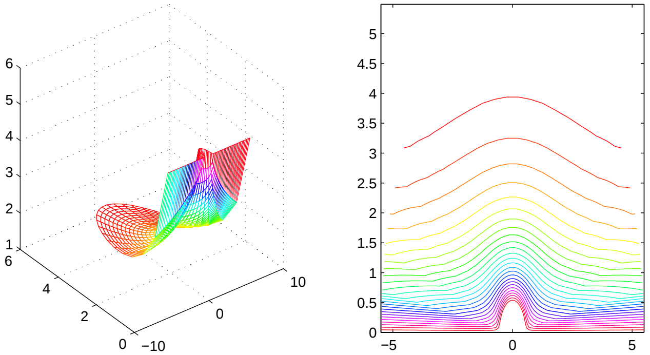
Figura 3.5: Dependência do campo magnético Meissner (a esquerda) e suas curvas de nível (a direita). Os parâmetros utilizados foram a = 0.5\lambda , \beta = \pi e H = 5 \frac{\phi_0}{\lambda^2} .
