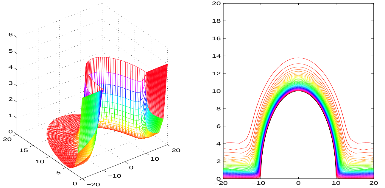
Figura 3.8: Campo Meissner de um supercondutor semi-infinito com uma indentação na presença de uma campo externo paralelo à superfície, no regime em que \lambda \ll a . Na esquerda temos o campo encontrado pela equação 3.46 e à direita suas curvas de nível. Os parâmetros utilizados foram : N = 1 , a = 10\lambda , \beta = \pi e H = 5\frac{\phi_0}{\lambda^2} .
