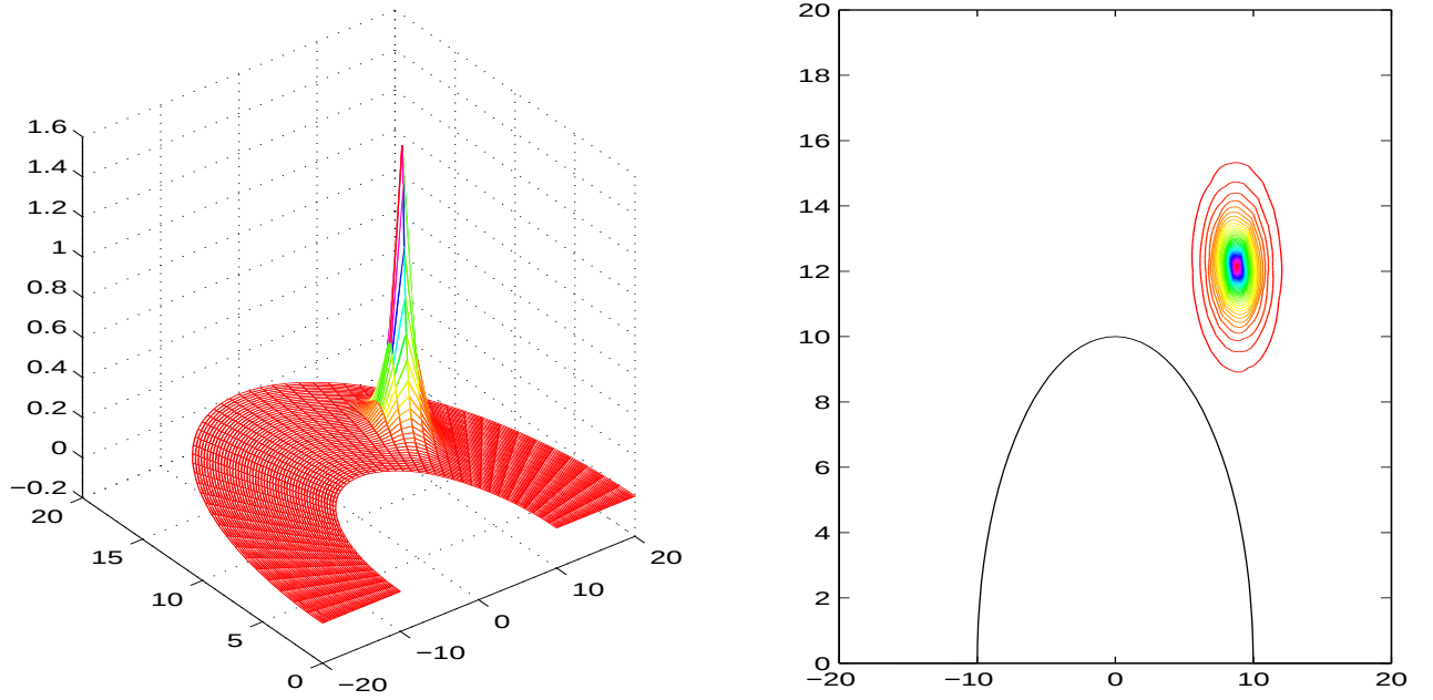
Figura 3.7: Auto-campo magnético em um supercondutor semi-infinito com uma indentação na superfície contendo um vórtice no interior no regime em que \lambda \ll a . À esquerda nós temos o auto-campo encontrado pelas equações 3.36 e à direita suas curvas de nível. Os parâmetros utilizados foram : N = 1 , a = 10\lambda e \beta = \pi .
