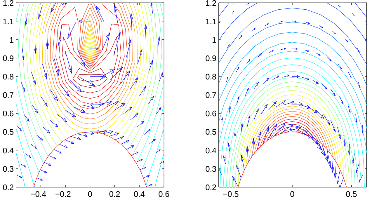
Figura 3.6: À esquerda nós temos o campo vetorial da densidade de corrente devido ao vórtice-antivórtice (Eqs. 3.25 e 3.26). Esta contribuição é devido ao termo h_1 . À direita nós temos o campo vetorial devido à indentação, (Eqs. 3.27 e 3.28). Esta contribuição é devido ao termo h_a . Os parâmetros utilizados foram a = 0.5\lambda , \rho_i = \lambda e \phi_i = \frac{\pi}{2} .
