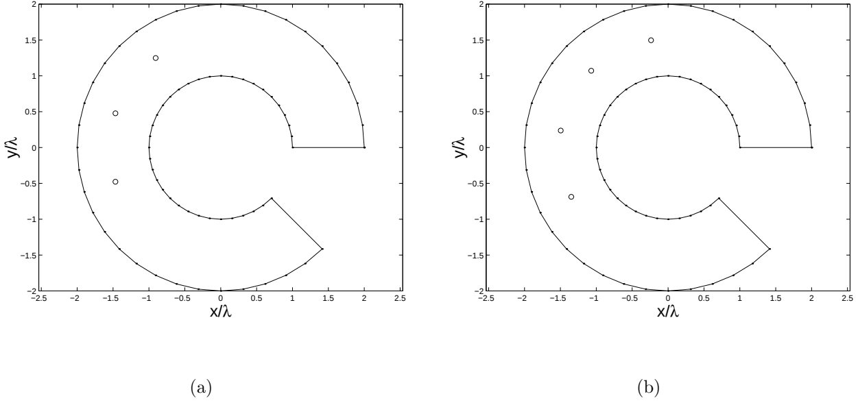
Figura 4.10: A medida que o ângulo \beta cresce, a geometria aproxima-se de um dispositivo SQUID. Os parâmetros utilizados foram: a = \lambda , b = 2\lambda e \beta = 1,8\pi
