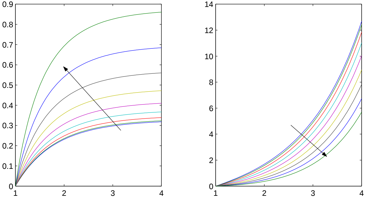
Figura 3.4: Gráfico das funções auxiliares. Dependência espacial de \Omega_m(y) (esquerda) e \Psi_m(y) (direita), para m=0, 0.25, 0.5, 0.75, 1, 1.25, 1.50, 1.75 e 2 . A seta indica o sentido do crescimento do índice m . As funções foram calculadas numericamente.
