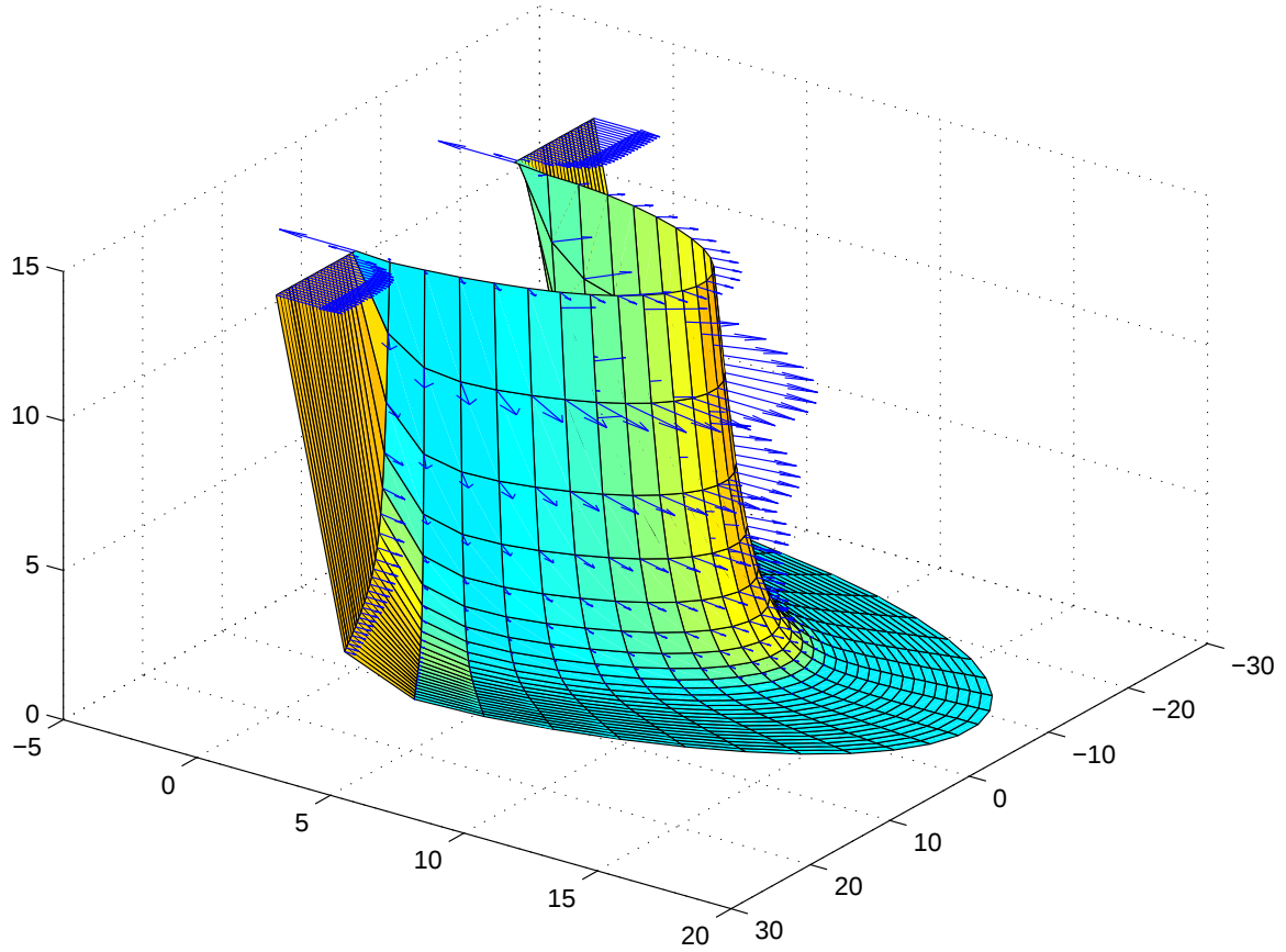
Figura 3.14: Força que atua sobre um vórtice dentro de um meio supercondutor semi-infinito com uma indentação na superfície. Os vetores da força sobre a superfície da energia após a força tornar-se positiva, ou seja, passar a atuar sobre um vórtice de forma a empurrá-lo para o interior do material. Os parâmetros envolvidos foram: a = \lambda e \xi = \lambda/60
